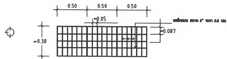
ฝาดะแครงเหล็กรางระบายน้ำ มาตราส่วน 1:25
