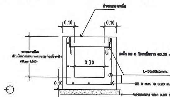
ฝาดะแครงเหล็กรางระบายน้ำ มาตราส่วน 1:25
