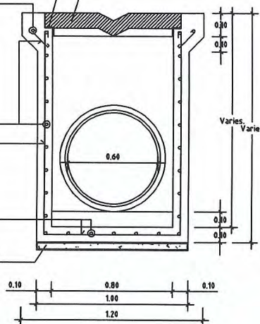
รูปตัดบ่อพัก คสล
